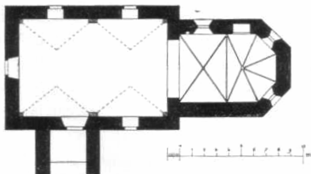
Obr. 109. Střížov. Půdorys kostela.
